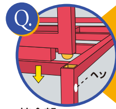
接合部
